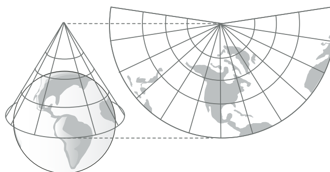
Proyección cónica
