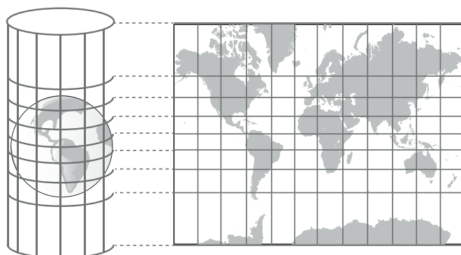
Proyección cilíndrica
