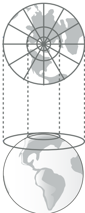
Proyección polar
